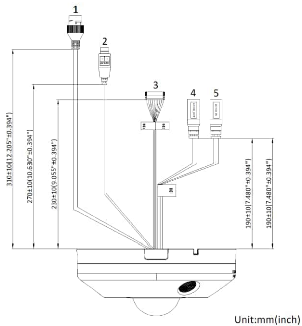
Unit:mm(inch)
