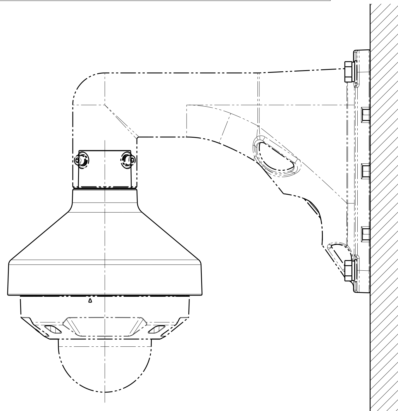
カメラとの組み合わせ例 Example of combination with a camera
