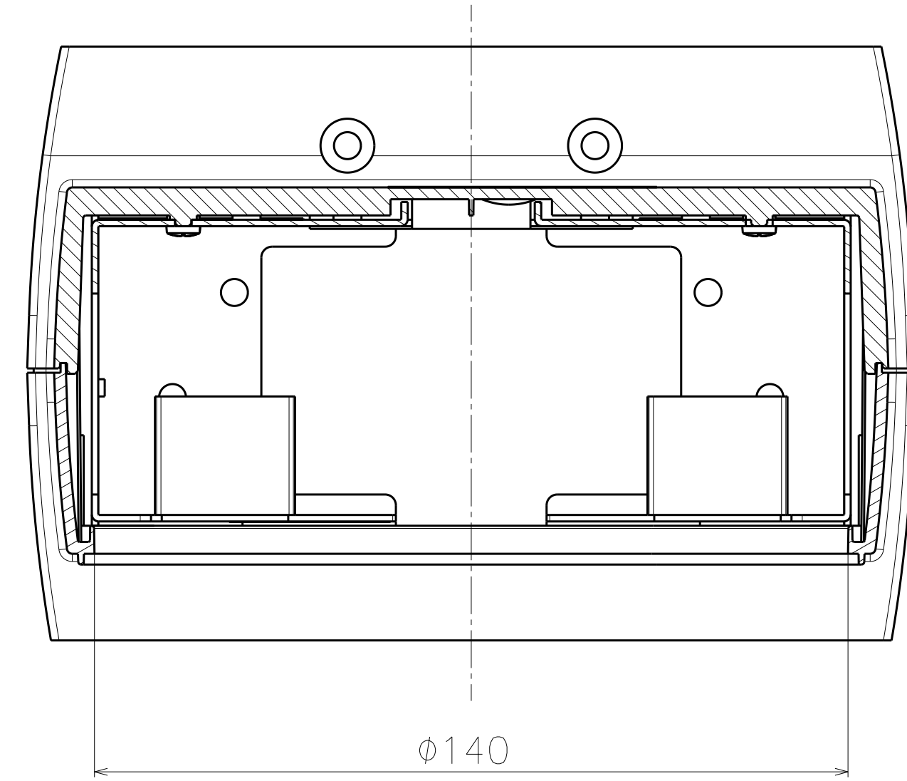
Sec A-A
