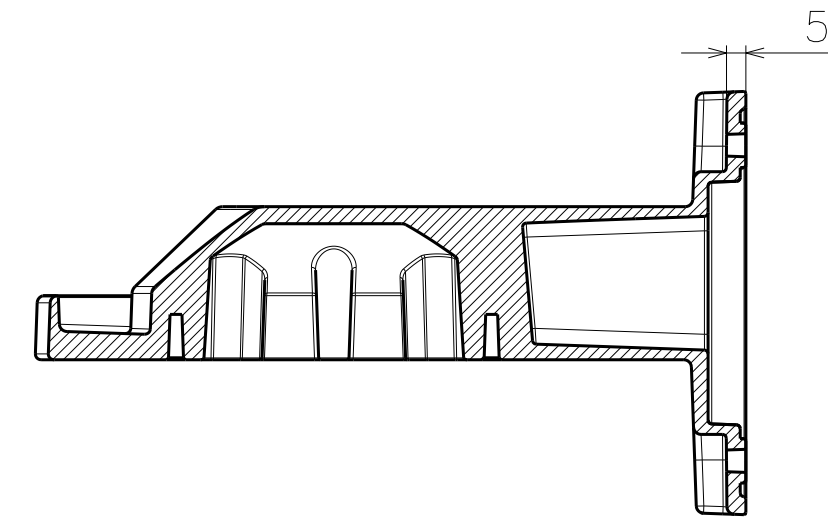
Sec A-A (1:2)
