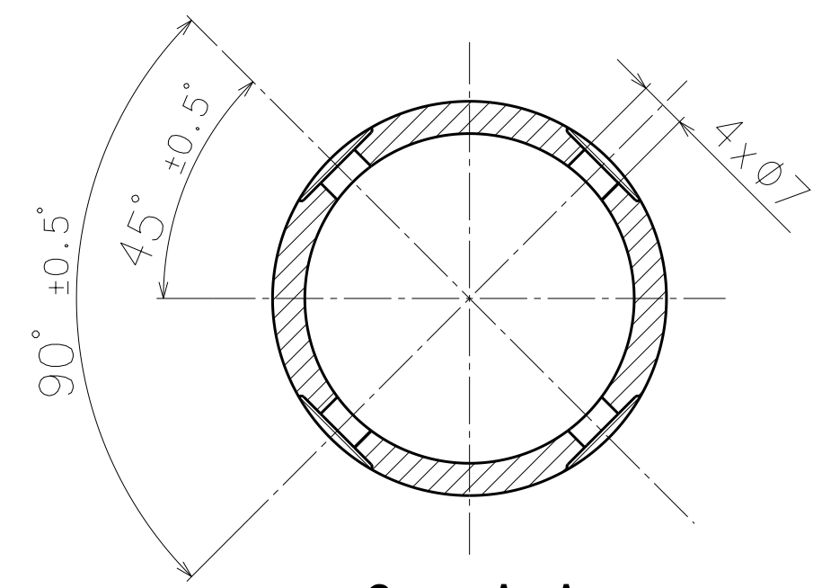
Sec A-A
