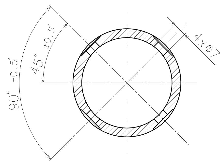
Sec A-A
