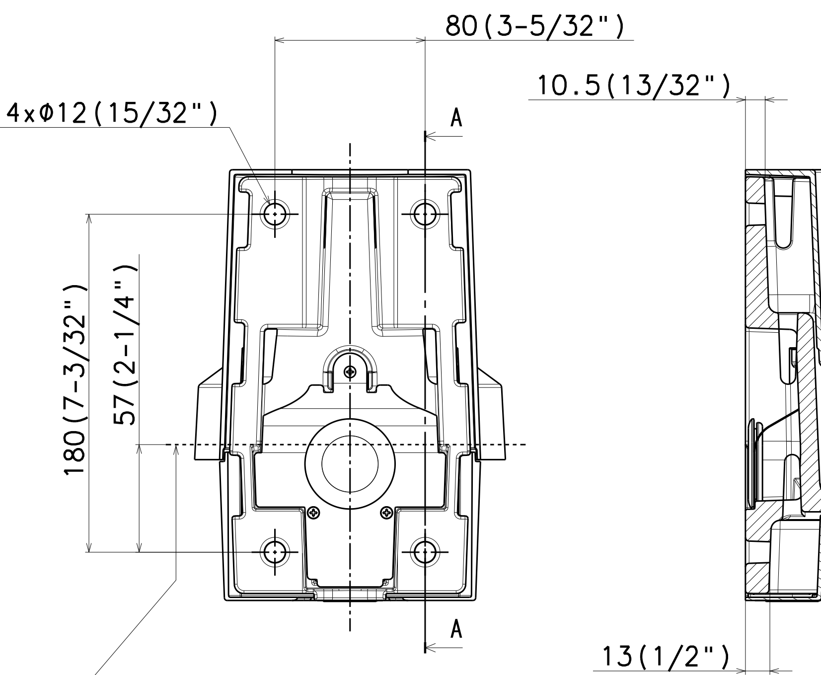
Sec A-A
