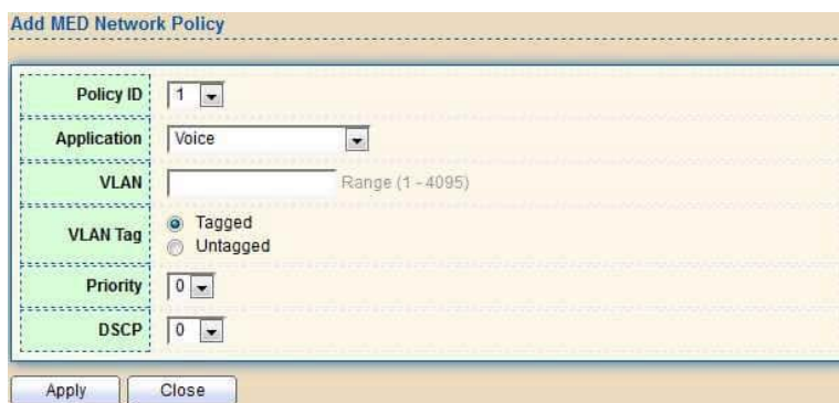
Figure 72 - Discovery > LLDP > MED Network Policy
